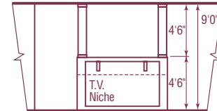
Elevation A - T.V. Niche
