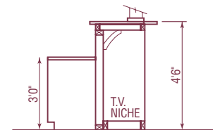
Elevation B - T.V. Niche
